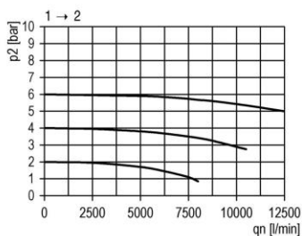
Durchflussdiagramm
